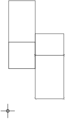
A: \langle U_{12} \rangle
