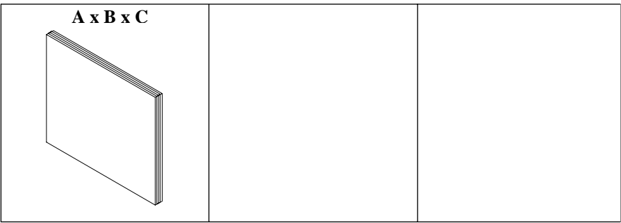
U_{23} \times U_{33} \times U_{33}
